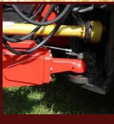
Ovládání nuceného řízení pomocí lanovodu
